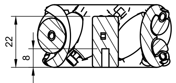
A-A (1:1)
